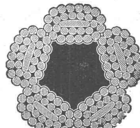
Patentiert „flachflitzige“ Drahtseile.
