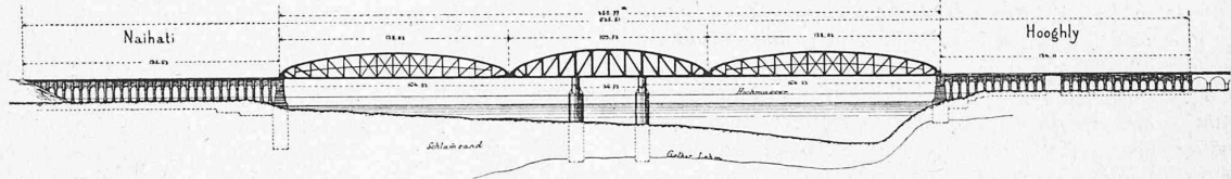
Fig. 2. Jubiläumsbrücke bei Hooghly in Ostindien. Gesamt-Ansicht.
