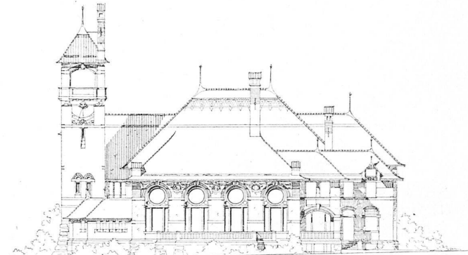
Südost-Ansicht 1 : 600.
