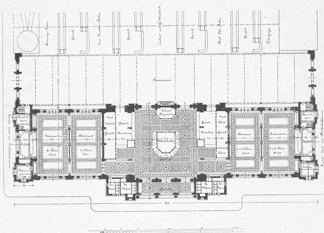
Grundriss.
