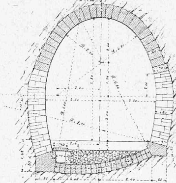
Nr. 5. Im Gebirge mit grossem Seitendruck.
