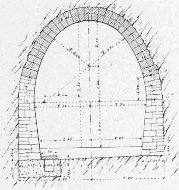
Nr. 4. Im Gebirge mit grossem Vertikaldruck.
