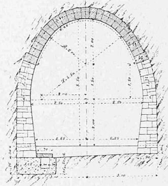
Nr. 6. An der Ausweichstelle (Tunnelmitte).
