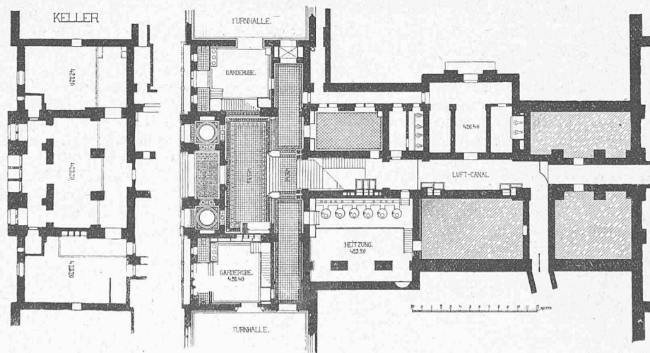
Kellergeschoss 1 : 500.
