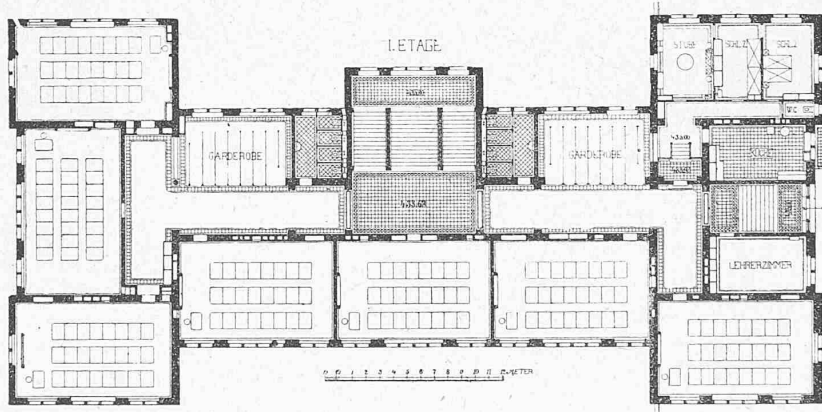
Grundriss vom ersten Stock.
