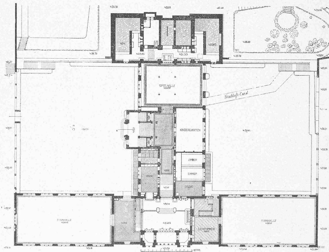
Lageplan und Grundriss vom Erdgeschoss.
