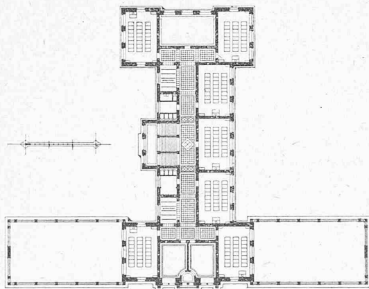
Konkurrenz-Entwurf Weinschenk. II. Preis.
