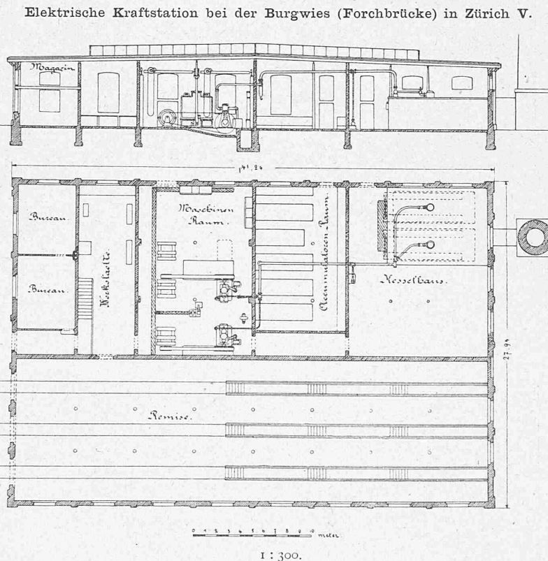
Fig. 3 und 4. Schnitt und Grundriss.
