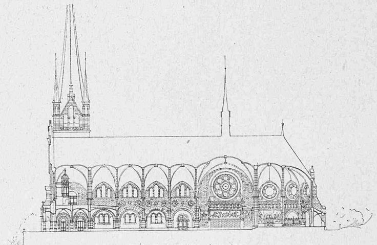
Längenschnitt 1 : 800.
