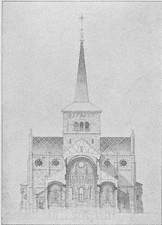
Querschnitt I : 800.
