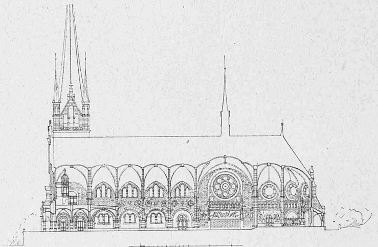
Längenschnitt 1 : 800.
