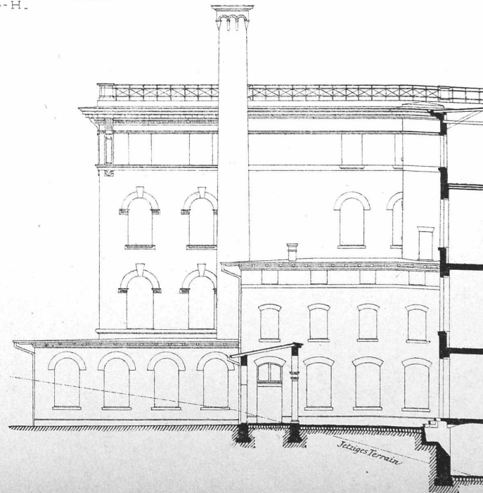
SCHNITT C-D
