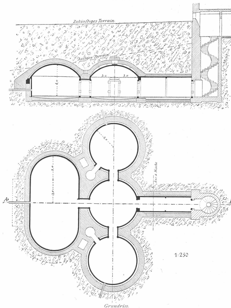
Grundriss.
