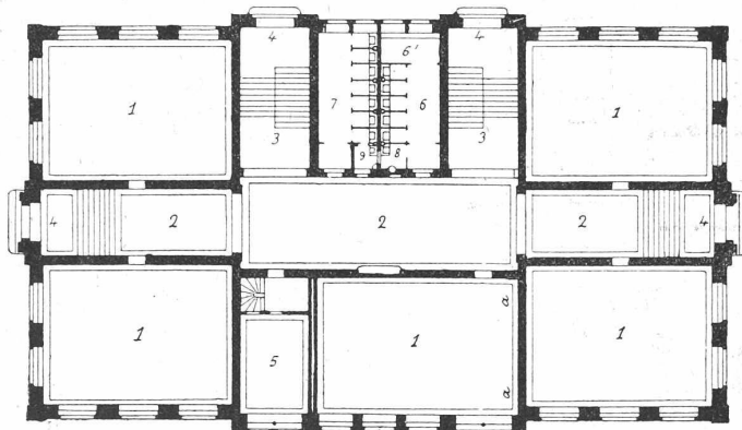
Grundriss vom Erdgeschoss.
