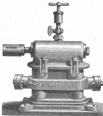
Bewährter Wassermesser zur Controlle der Dampfkessel. (M 1474 Z) Medaille d'honneur de la Société industrielle de Mulhouse 1885.
