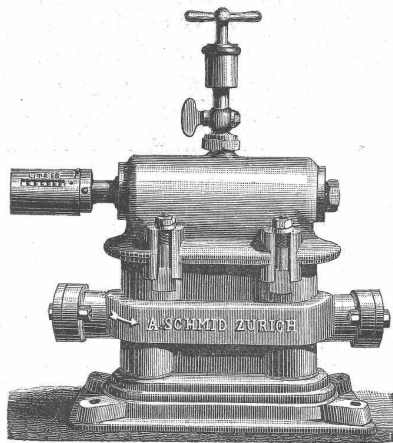
Bewährter Wassermesser zur Controle der Dampfkessel.
