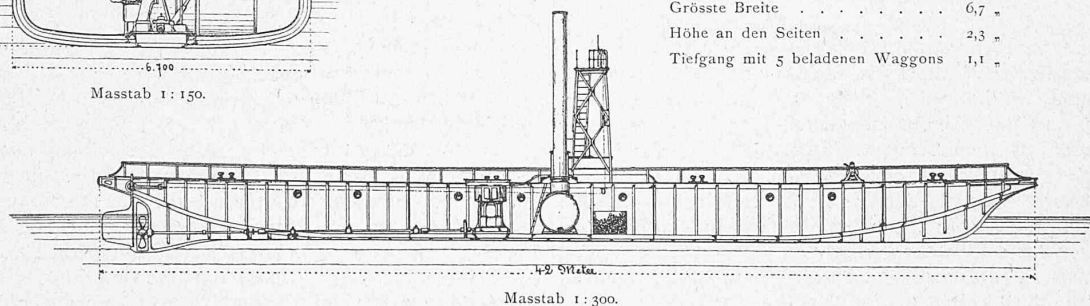
Längsschnitt.
