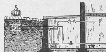
Hausverbindungen.
