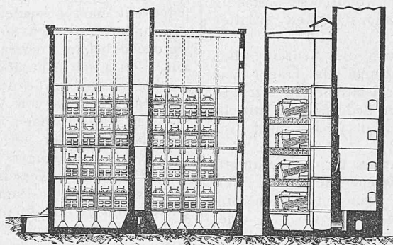
Längenschnitt.
