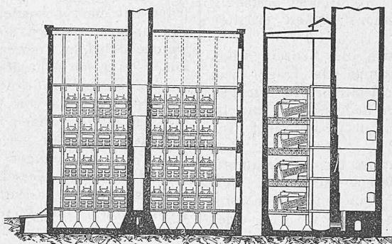
Längenschnitt.
