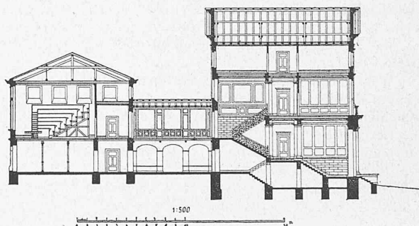
Schnitt.
