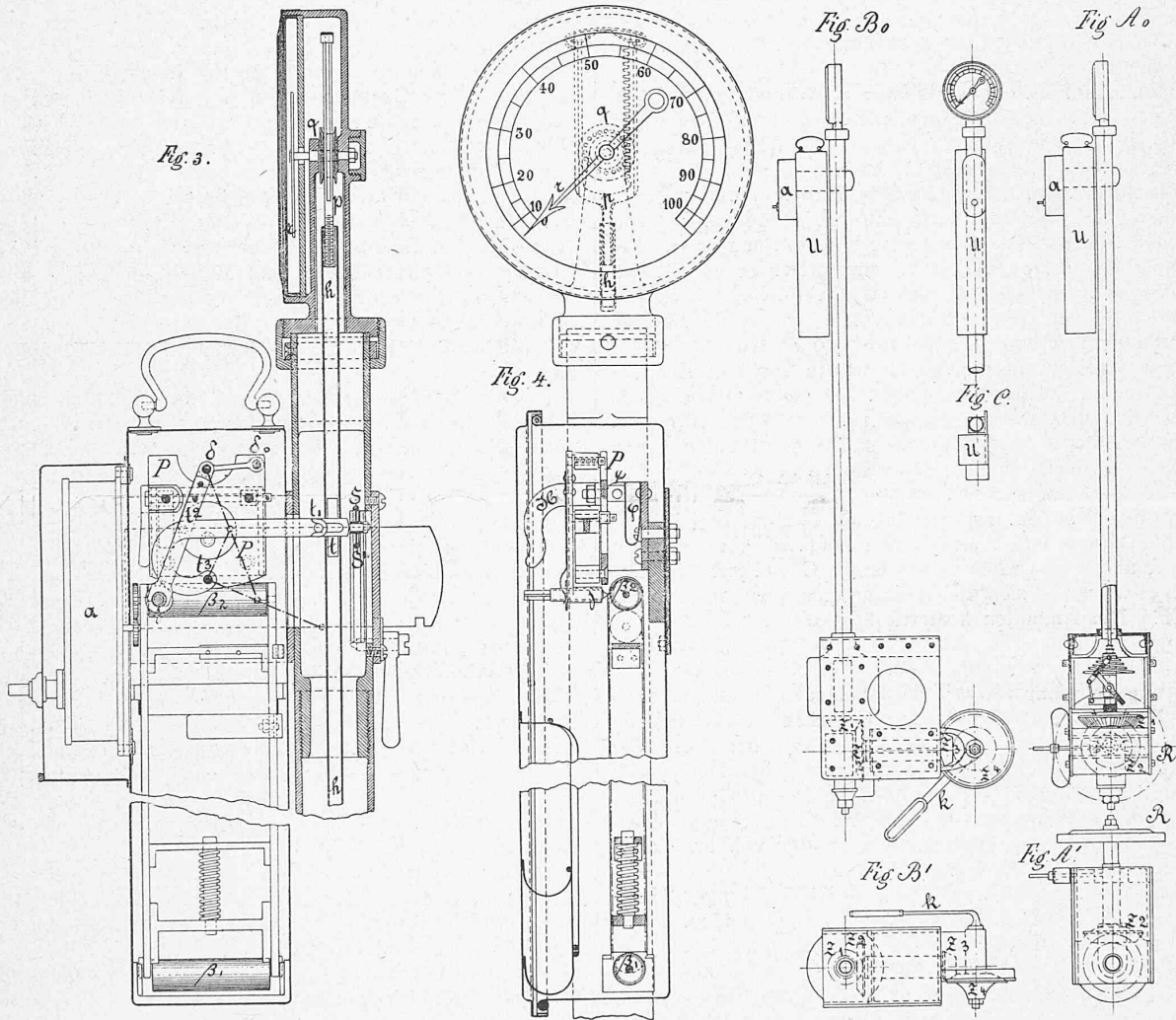
Gesamtansicht. Masstab 1 : 20.
