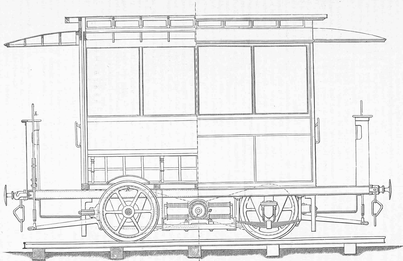
Fig. 13. Wagen der electricen Eisenbahn in Lichterfelde von Siemens & Halske in Berlin. Längs-Ansicht und -Schnitt. Masstab 1 : 25.
