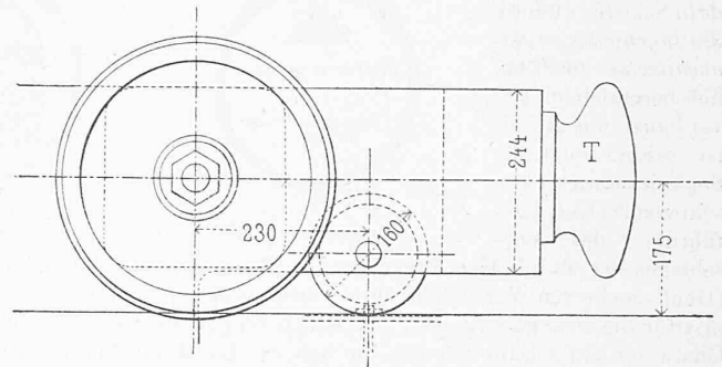
Aufriss des Wagens. — Masstab 1 : 10
