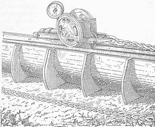
Perspektivische Ansicht des Wagens und des Rohres
