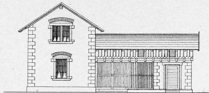
Ansicht gegen die Bahn
