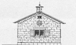
Ansicht gegen die Bahn
