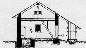
Schnitt A.B
