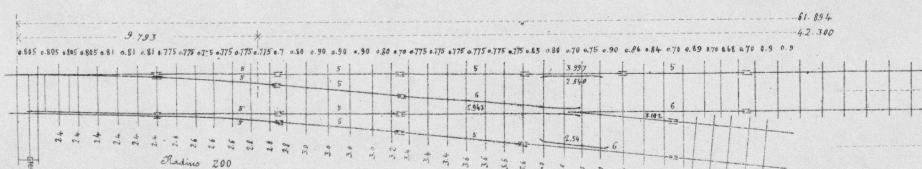
Rechtsweiche für Hauptgleise Tangente 1:9
