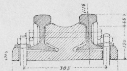
Schnitt II. 1:9
