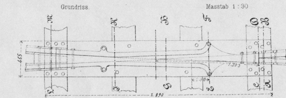
Gussstahl-Herzstück Kreuzungs-Tangente 1:11
