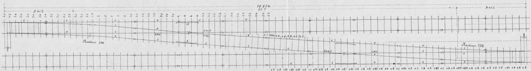
Endweiche für Bahnhöfe Kreuzungs-Tangente 1:11
