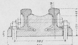
Schnitt II. 1:9
