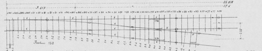
Rechtsweiche für Nebengleise Tangente 1:8
