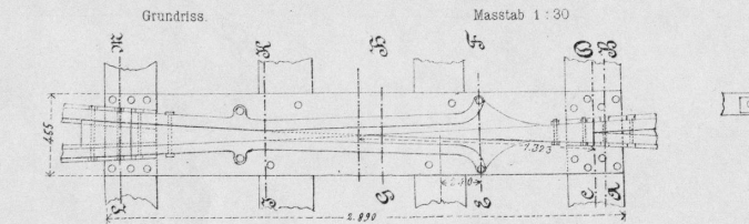
Gussstahl-Herzstück Kreuzungs-Tangente 1:11
