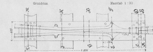
Gussstahl-Herzstück Kreuzungs-Tangente 1:11
