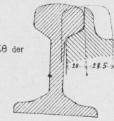
gebogenen Zunge
