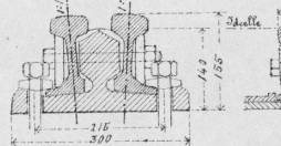
Schnitt III. 1:9
