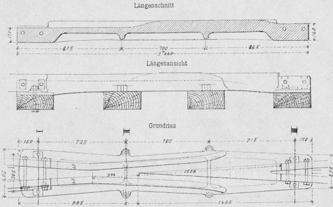
Gussstahl-Herzstück Kreuzungs-Tangente 1:11
