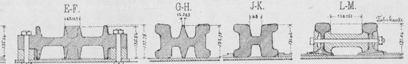
Querschnitte des Gussstahl-Herzstückes Masstab 1:10
