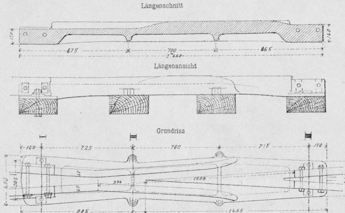
Gussstahl-Herzstück Kreuzungs-Tangente 1:11
