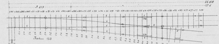
Rechtsweiche für Nebengleise Tangente 1:8
