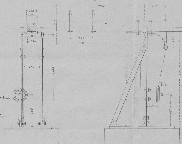
Fig. 4. Seitenansicht.
