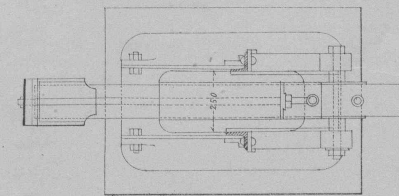
Fig. 9. Grundriss
