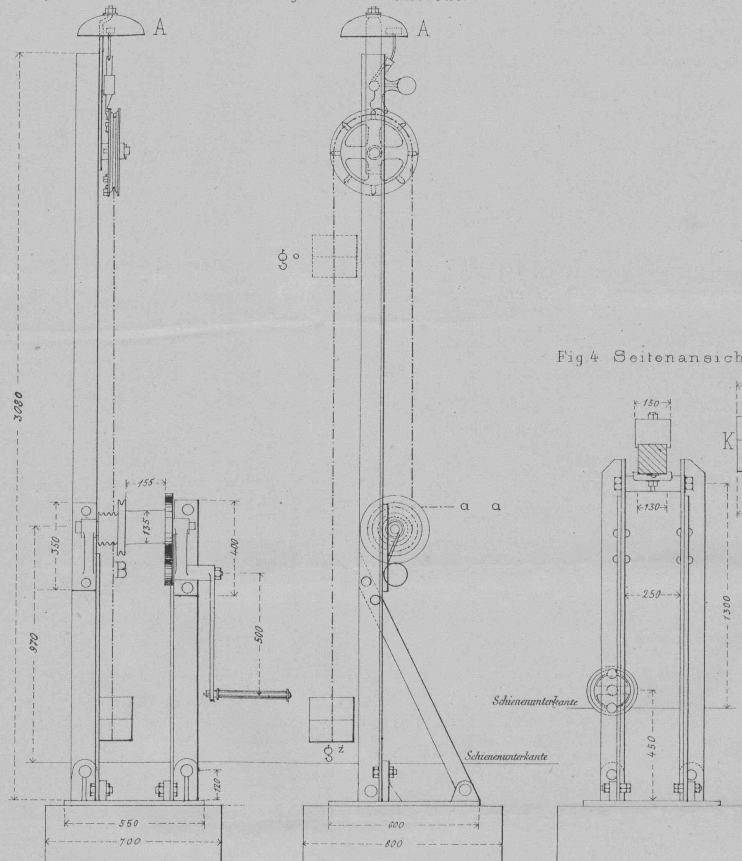
Fig. 1. Seitenansicht
