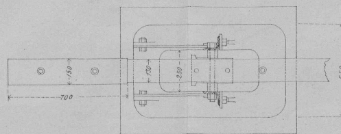
Fig. 6. Grundriss
