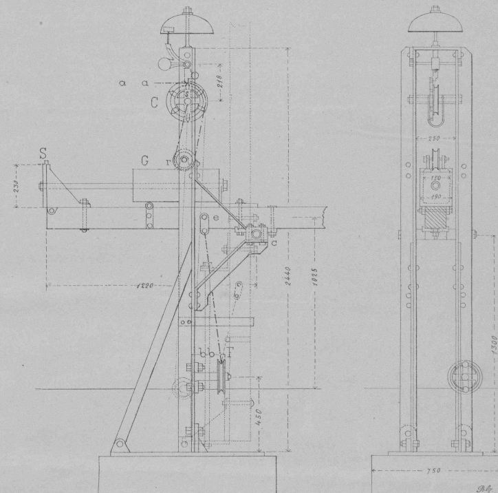
Fig. 7. Vorderansicht
