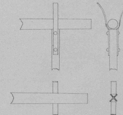
Schlagbaumträger
