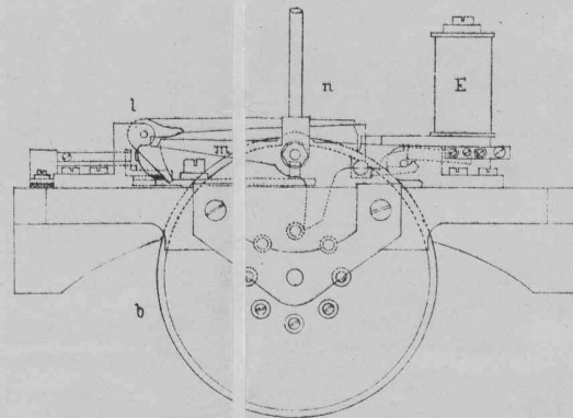
Fig. 4. Seitenansicht
