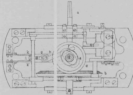
Fig. 3. Grundriss
