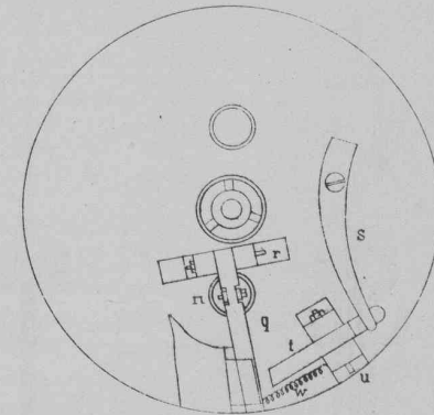
Fig. 5. Grundriss
