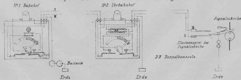
Fig. 7. Schema der Drahtverbindungen
