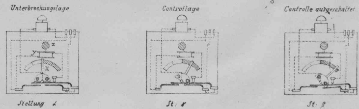
Controllkasten N o 1. mit verschiedenen Stellungen
