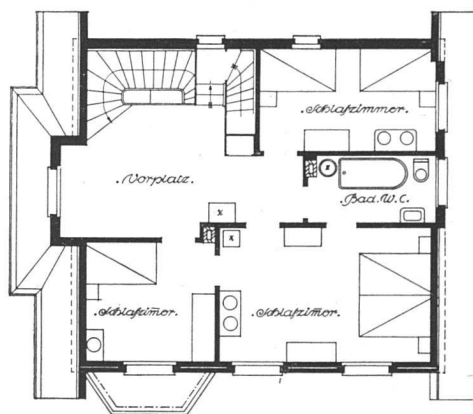
Wohnhaus von Ing. W. Haeberli-Walter in Balsthal. — Grundrisse. Links: Erdgeschoss. Rechts: Obergeschoss. Masstab 1 : 200 Architekten von Arx & Real, Olten.
