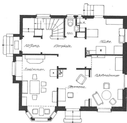
Wohnhaus von Ing. W. Haeberli-Walter in Balsthal. — Grundrisse. Links: Erdgeschoss. Rechts: Obergeschoss. Masstab 1 : 200 Architekten von Arx & Real, Olten.
