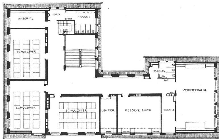
Schulhaus in Kolliken. — Grundriss vom zweiten Stock. Masstab 1 : 400
