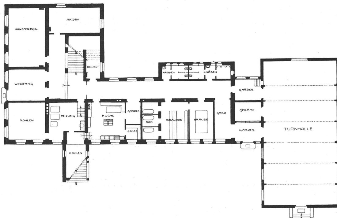
Schulhaus in Kölliken. — Grundriss vom Untergeschoss.
