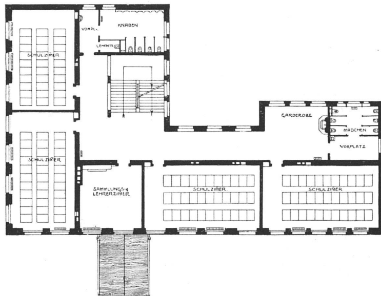
Schulhaus in Kolliken. — Grundriss vom ersten Stock. Masstab 1 : 400
