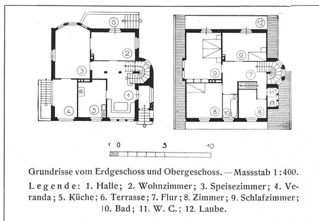
Wohnhaus des Herrn Hans Stücklin-Amapane an der Wenkenhalde in Riehen bei Basel.
