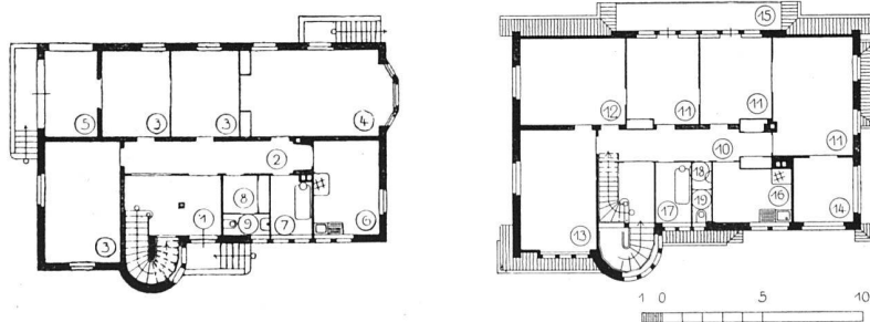
Grundrisse vom Erdgeschoss und Oberstock. — Massstab 1:400.
