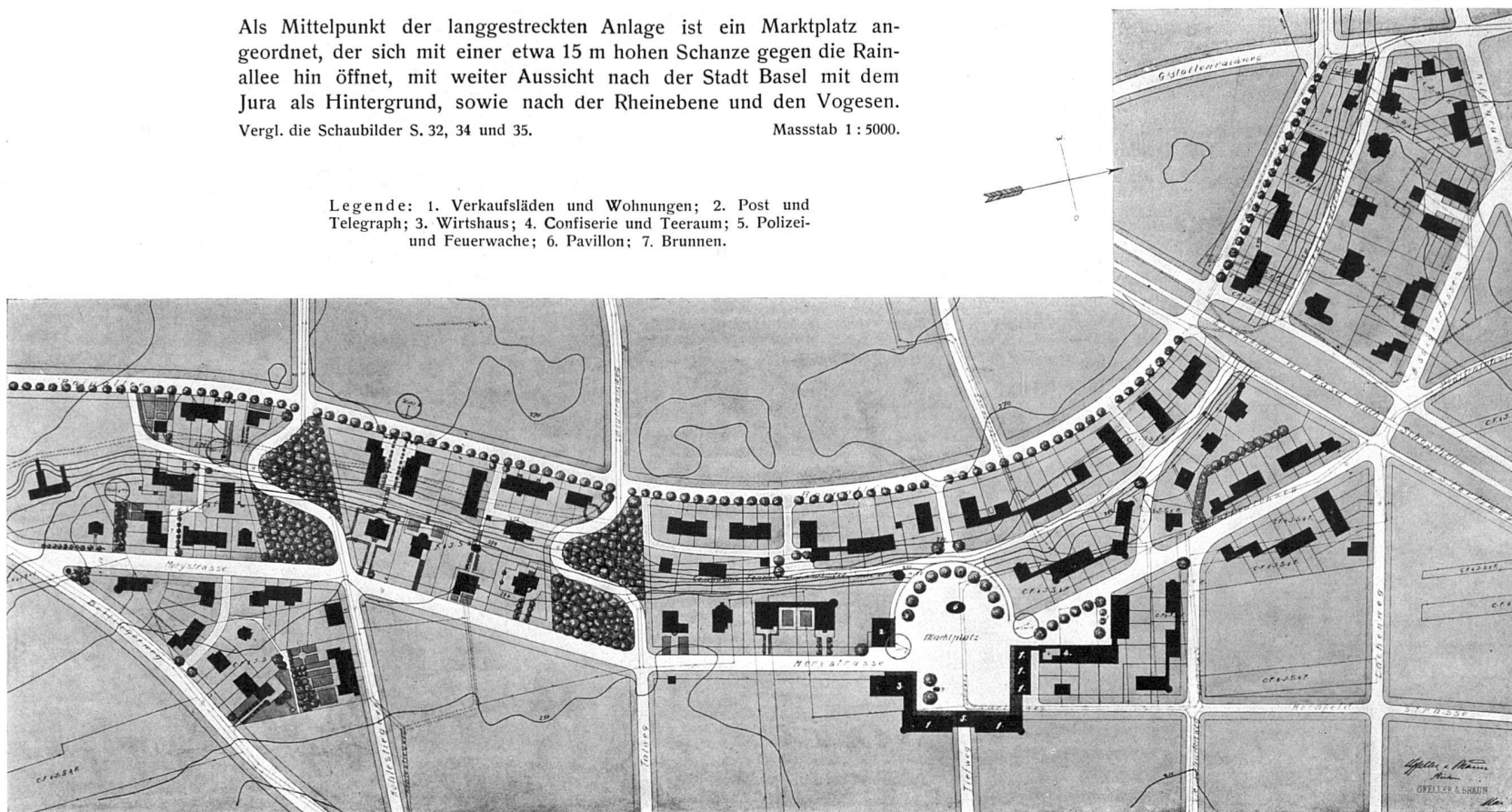
Uebersichtsplan des Entwurfs für die Ueberbauung des Geländes der Tit. Comp. Foncière et Immobilière Suisse et Française zu Riehen. Architekten Gfeller & Braun, Riehen bei Basel.
