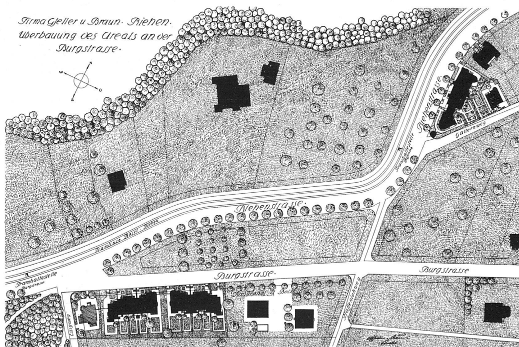
Uebersichtsplan über die Ueberbauung der Gelände an der Burgstrasse, der Riehenstrasse und dem Gatternweg in Riehen bei Basel. — Massstab 1 : 2500. Architekten Gfeller & Braun, Riehen bei Basel.
