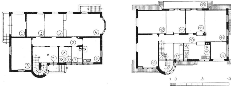
Grundrisse vom Erdgeschoss und Oberstock. — Massstab 1:400.
