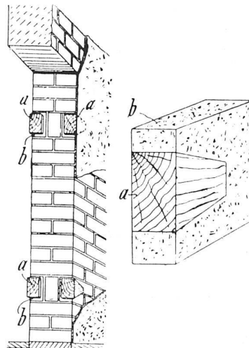
Eingegossener Holzdübel.
