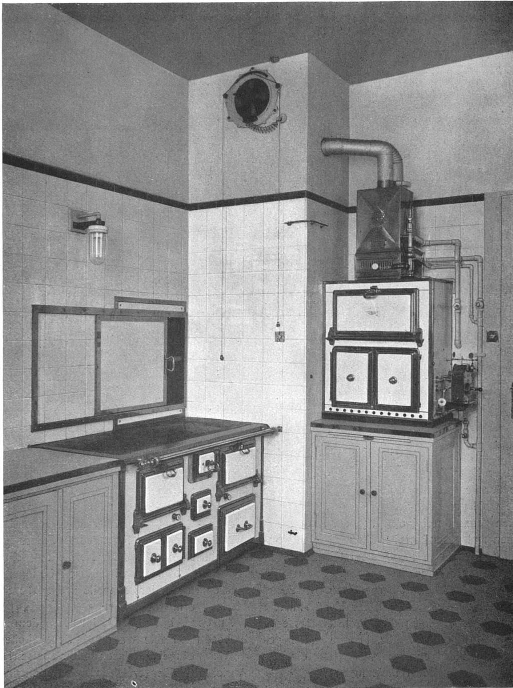
Aus der Küche der Villa Wegelin-Hauser in St. Gallen. Senking Kohlenherd, darüber Wärmeschrank, daneben Heisswasserapparat und kombinierte Spiess- und Grill-Einrichtung mit Backofen.
