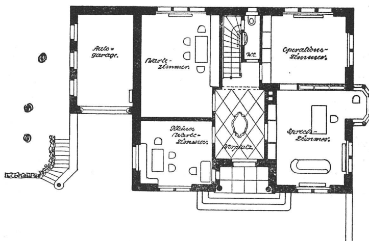
Erdgeschoss-Grundriß Maßstab 1:200
