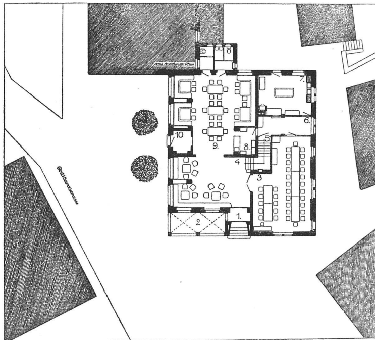
Erdgeschoss-Grundriß und Situation Maßstab 1:400
