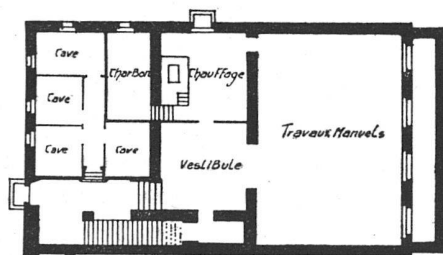
Kellergeschoss
