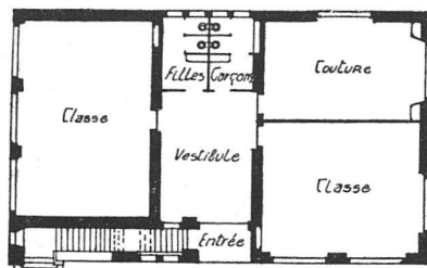
Erdgeschoss
