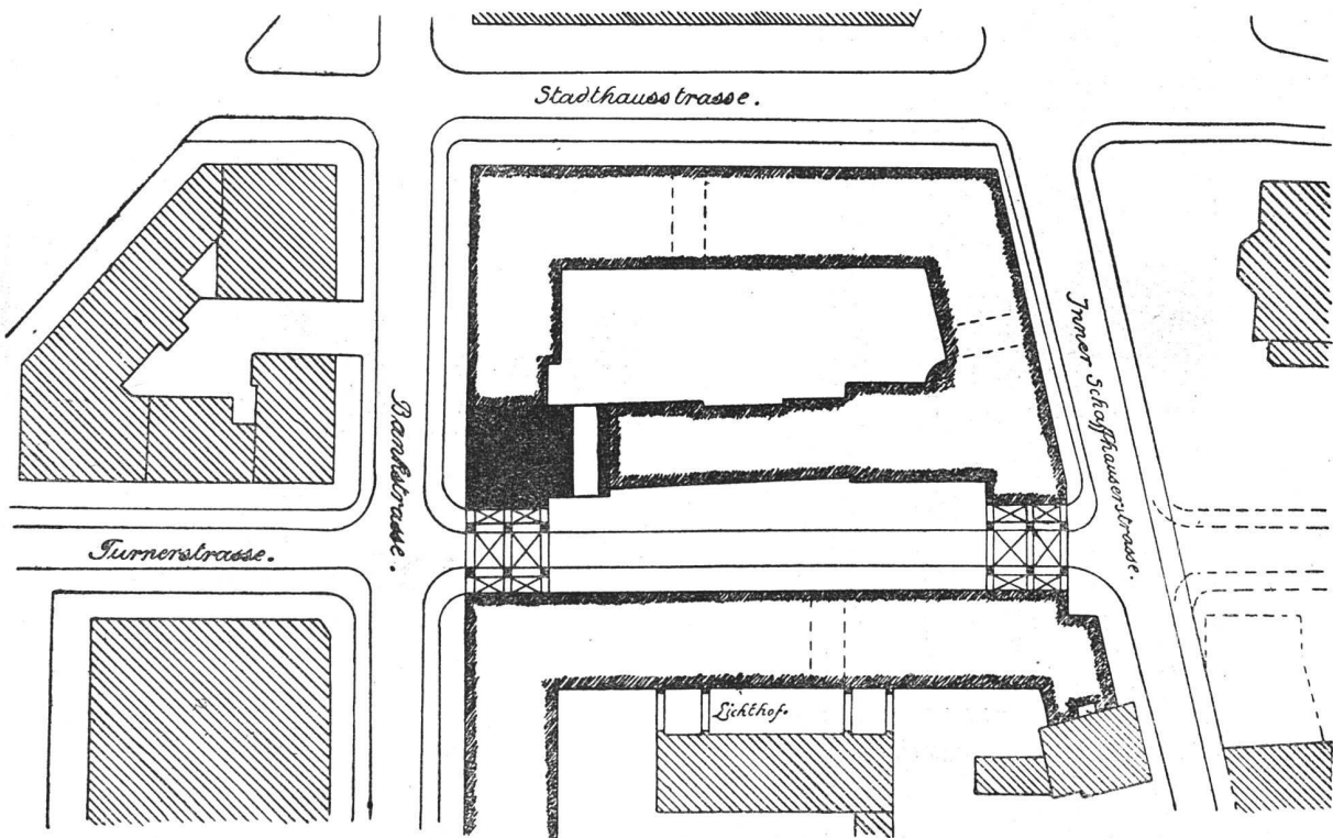
Gesamtlageplan 1:1000
