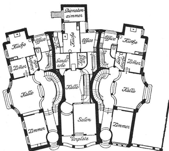
Grundriß des Erdgeschosses 1:400
