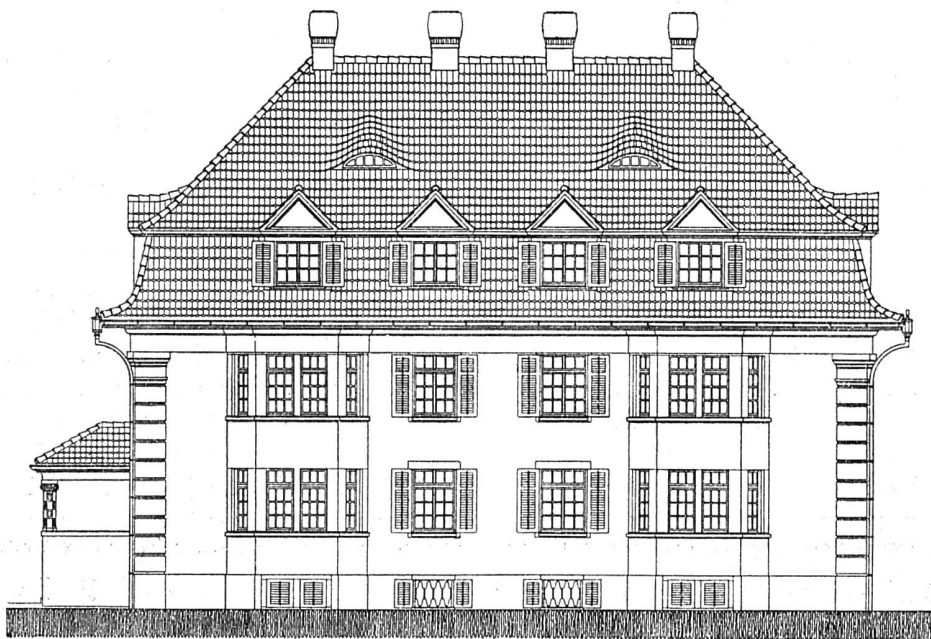
Das Pfarrhaus in Auserzhofen. — Architekten (B. S. A.) Gebrüder Braem in Zürich. — Hauptfassade. — Maßstab 1:200
