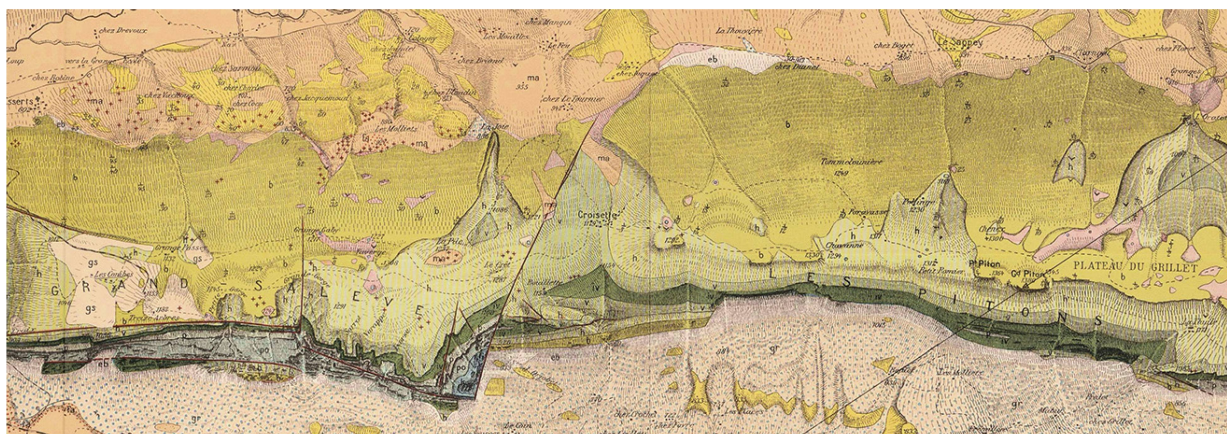
Fig. 9. Carte géologique du Grand Salève aux Pitons. En jaune-vert, noté m , les calcaires urgoniens; en vert acide, noté h , les calcaires hauteriviens. En bleu clair et foncé, notés po et k , les calcaires jurassiques. (J&F, 1913).
