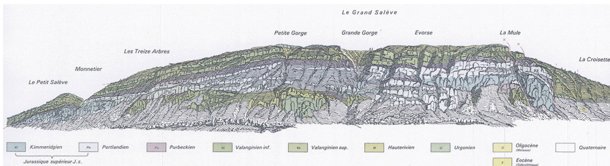
Fig. 3. Le Petit Salève (à gauche) et le Grand Salève, vus de Troinex, dessinés par A. Lombard. Les vallons perchés - la Petite et la Grande Gorge - ainsi que le vallon sous La Mule, sont entaillés à l'extrémité d'accidents mineurs (failles) recoupant le massif perpendiculairement à son axe. A partir de la Petite Gorge, les bancs s'inclinent vers le NE (à gauche) avec un pendage de 8° au droit de Monnetier (LOMBARD, 1965).
