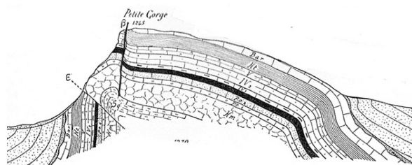
Fig. 4. Coupe du Salève au niveau de la Petite Gorge, telle que reconstituée par J&F (1913). La strate en noir repère le Purbeckien, un niveau d'eau douce à plantes, dont des Chara , ancêtres des formes actuelles qui peuplent les mares sommitales.
