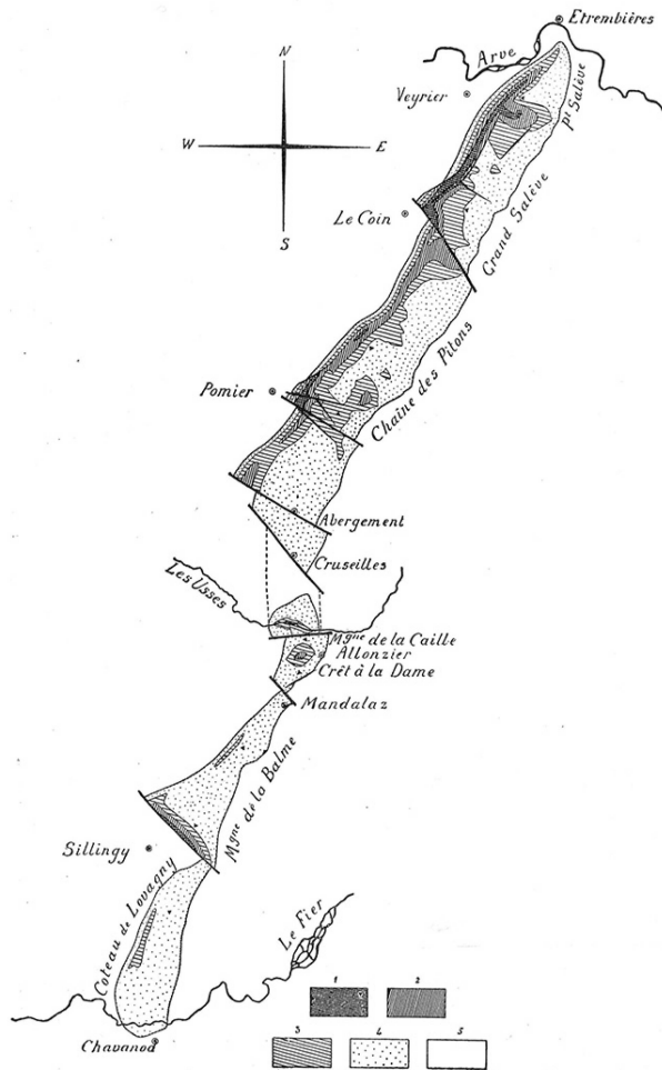
Fig. 6. Carte structurale du Salève avec les positions et orientations des décrochements (traits épais). Code des terrains : 1 : Jurassique ; 2 : Valanginien ; 3 : Hauterivien ; 4 : Barrémien et Aptien ; 5 : Tertiaire et Quaternaire. (J&F, p. 360). Echelle : 1 : 270'000.
