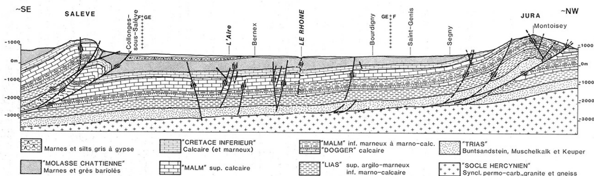
Fig. 5. Coupe du bassin genevois, du Salève (Les Pitons) à la Haute-Chaîne du Jura (Recullet). La structure profonde du Salève est une réplique de celle du chaînon le plus récent du Jura, avec décollement de l'ensemble de la série sédimentaire sur les couches plastiques à la base du Trias (anhydrite et sels). La fracturation et le repliement de l'avant de la lame glissée simulent des structures anticlinales. (AMBERGER, 1982).
