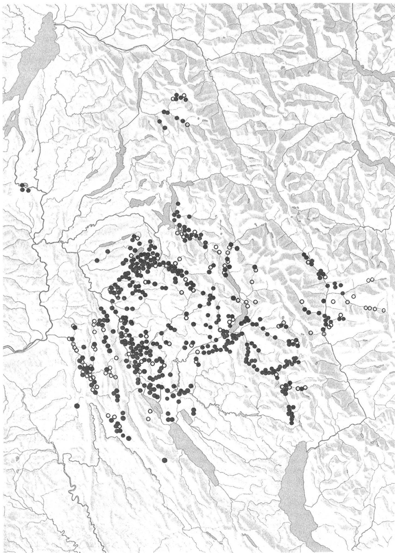
Abb. 1: Serologische Untersuchung auf RSV, geografische Verteilung der positiven (●) und negativen (○) Befunde
