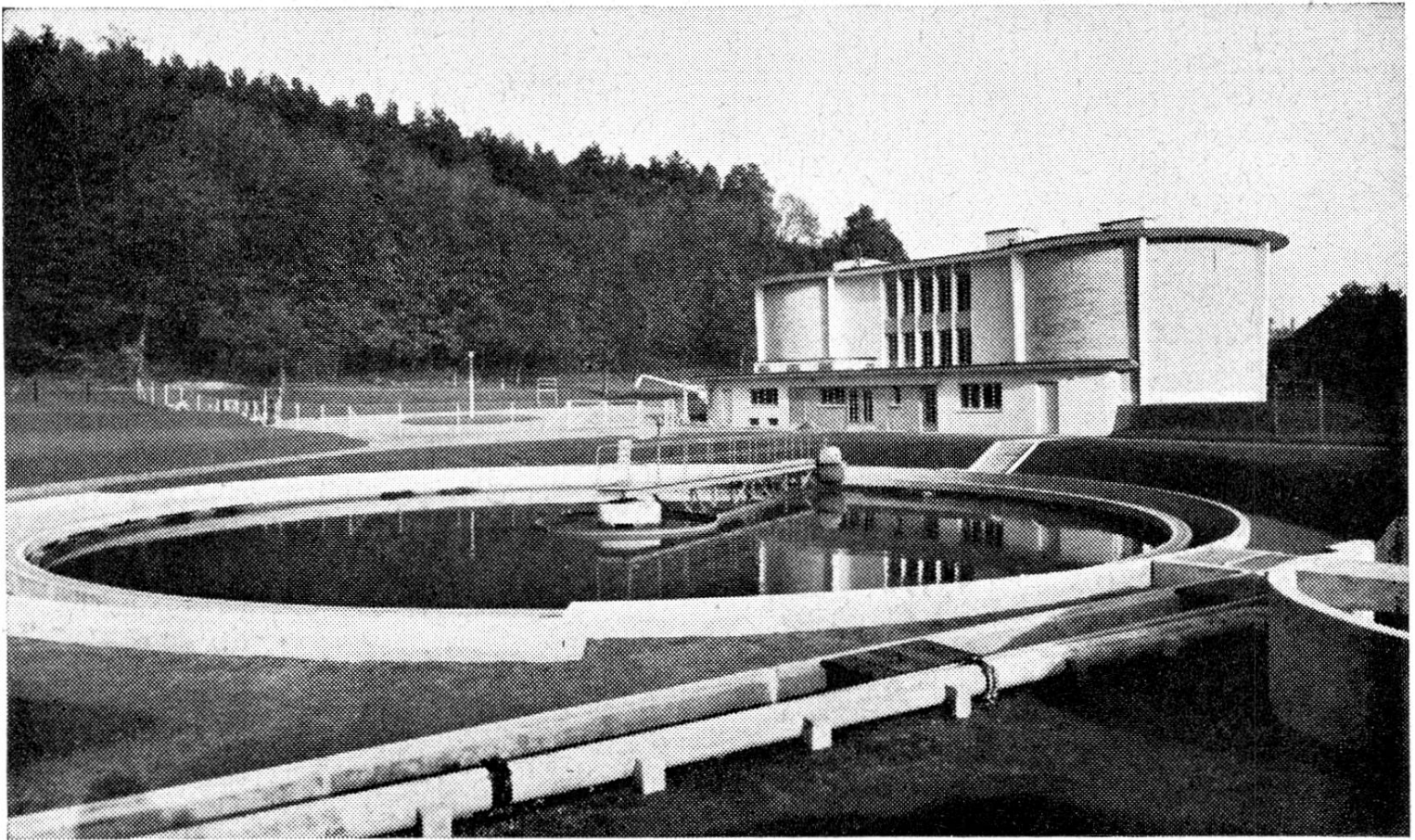
Abb. 2. Vorklärbecken, Schlammsfäulturne.
