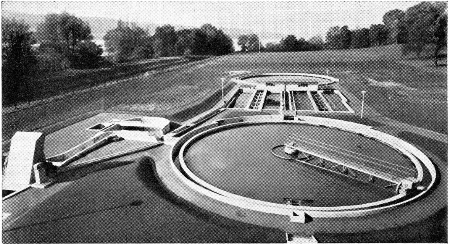
Abb. 1 1 . Mechanisch-biologische Kläranlage von Uster: Im Vordergrund: Klärbecken mit langsam sich drehendem, zeigerartigem Ölfang; dahinter erkennt man die doppelt angelegten Belebtschlammbecken (mit Metallbürsten) und ganz zu hinterst das Nachklärbecken.
