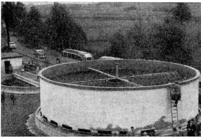
Abb. 3. Tropfkörper.
