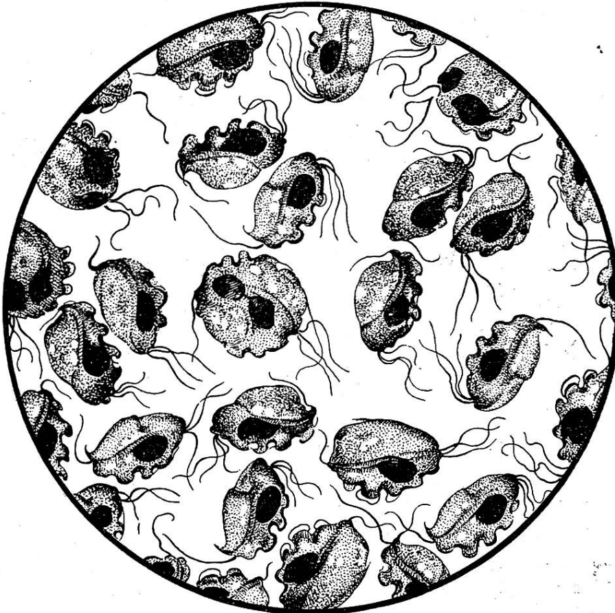
Trichomonas foetus
