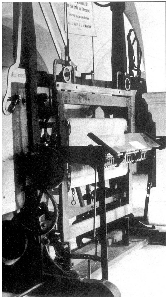
Technischer Quantensprung, der der Stickereibranche den Übergang zur Massenproduktion ermöglichte: Schifflistick-Maschine nach Plänen von Isaak Gröbli, erbaut von der Firma J. J. Rieter & Cie., Winterthur. Bilder: Archiv Hans Amann
