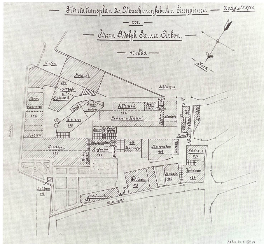
Situationsplan der Maschinenfabrik u. Eisengiesserei von Herrn Adolph Saurer Arbon, 8. Okt. 1903 Quelle: historisches Lexikon der Schweiz, E. Trösch, Buch Saurer, H.U. Wipf; M. König; A. Kneopfli
