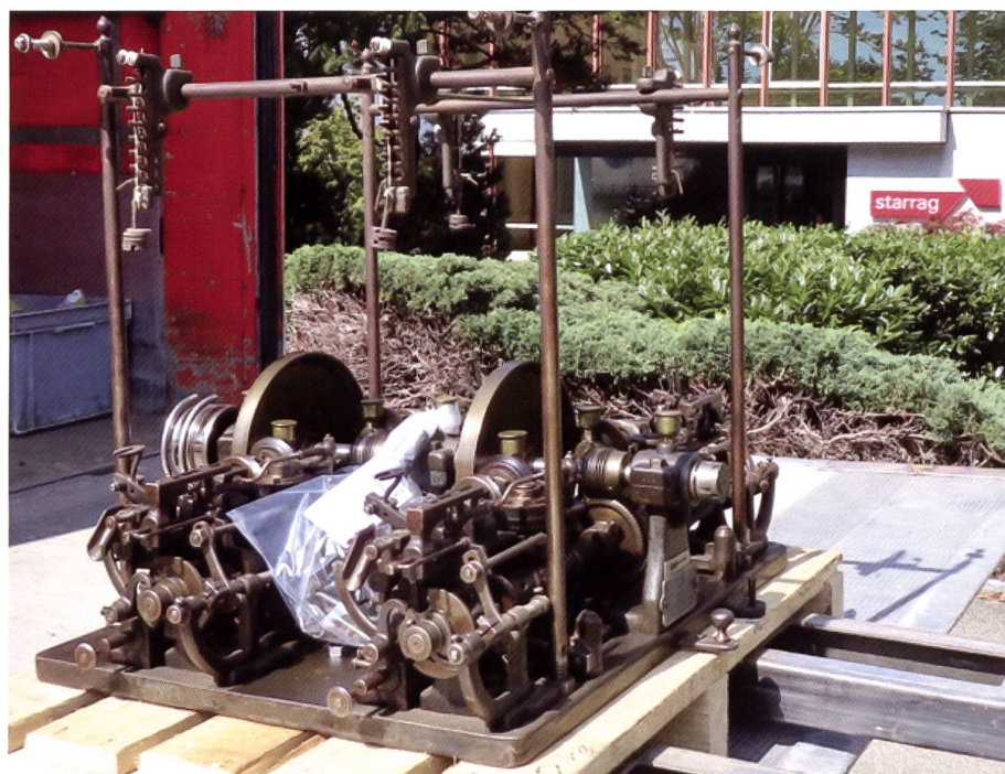
4-fach Bobinenmaschine mit Reibrad-Antrieb
