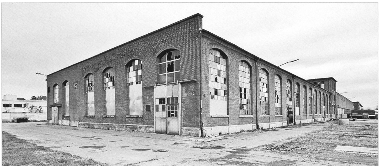
Den vorderen, grösseren Teil der Halle des alten Saurer-Presswerks bis zum Kopfbau (rechts) wird der Oldtimer Club Saurer als Schaulager nutzen. Im Vordergrund die lastwagentaugliche Einfahrt. HRS Renovation AG wird die ganze Gebäudehülle sanieren. Die östlich an den Kopfbau angebauten Gebäude (im Hintergrund) sollen dem neuen Hotel WerkZwei weichen. (Text und Bild: Max Eichenberger)
