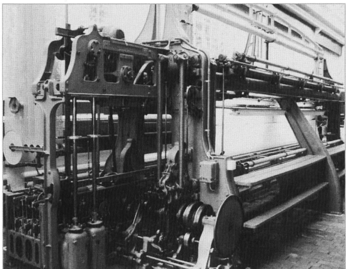
lochkartengesteuerte-Schiffli-Stickmaschine
