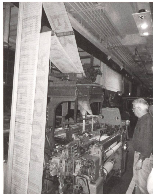
Die Webmaschine 100 WT Nr. 81426 an ihrem neuen Einsatzort. Und sie webt! Links die Lochkarte für die Aufschrift.
