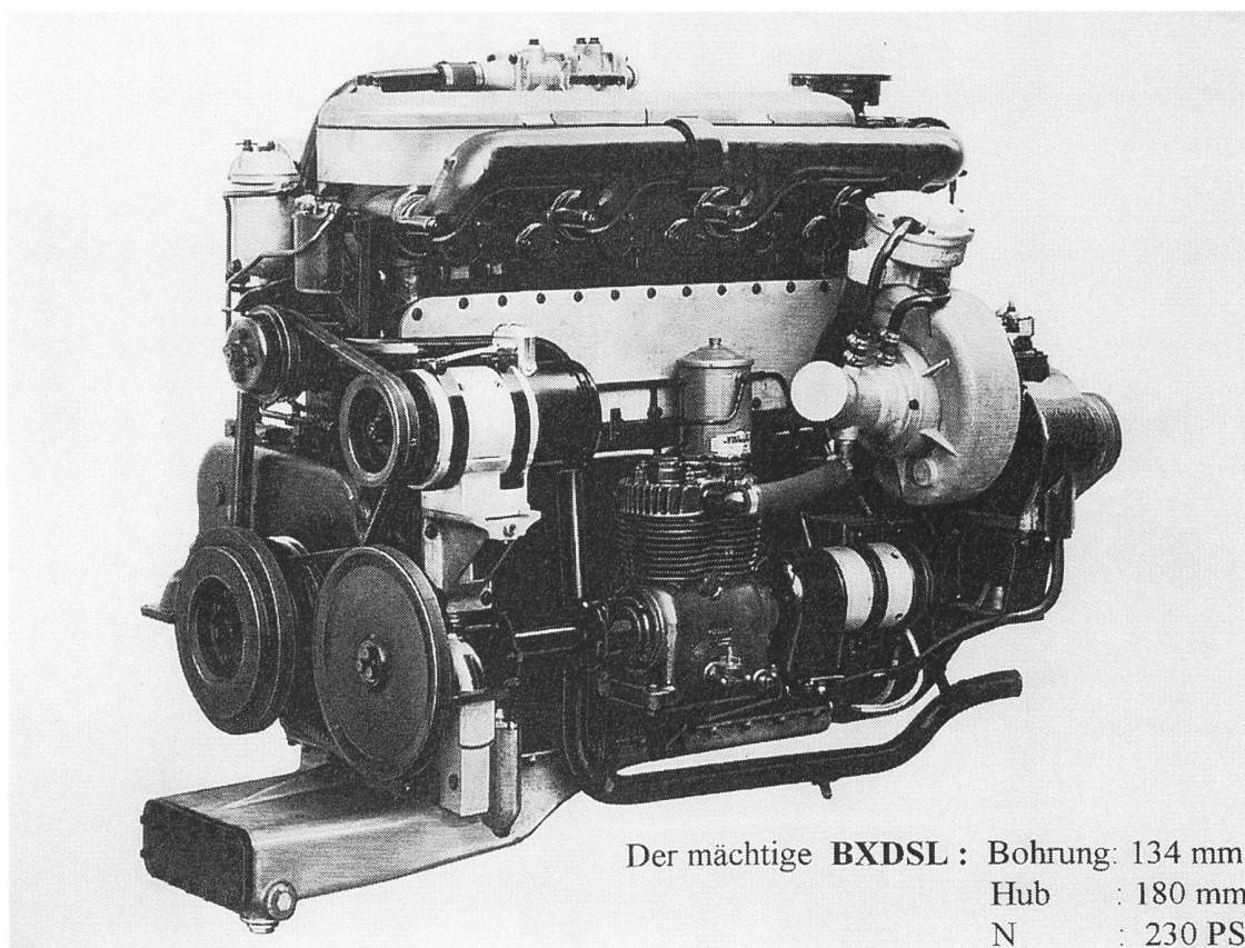
Versuchsfahrten für die Chilenischen Staatsbahnen auf der Linie Chur-Arosa. Insert: BXDSL mit Schleuderradgebläse
