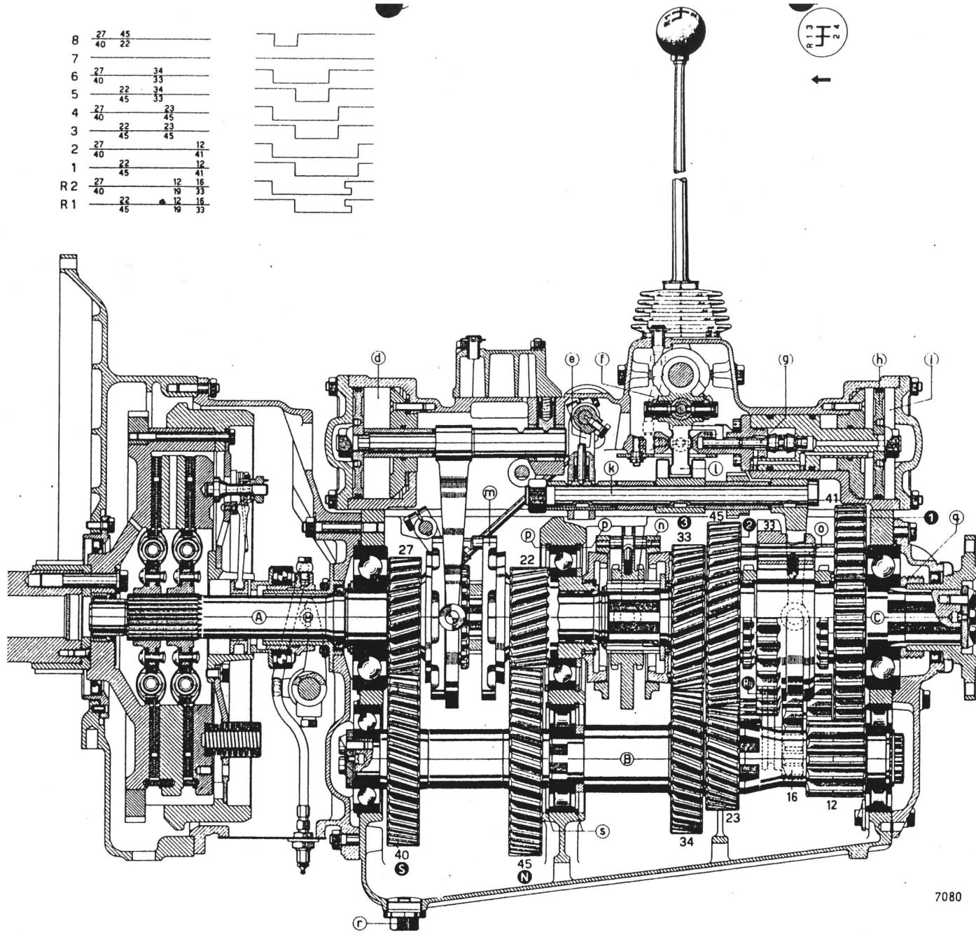
Schnitt durch das Achtgang-Servo-Handschaltgetriebe mit Kupplung
