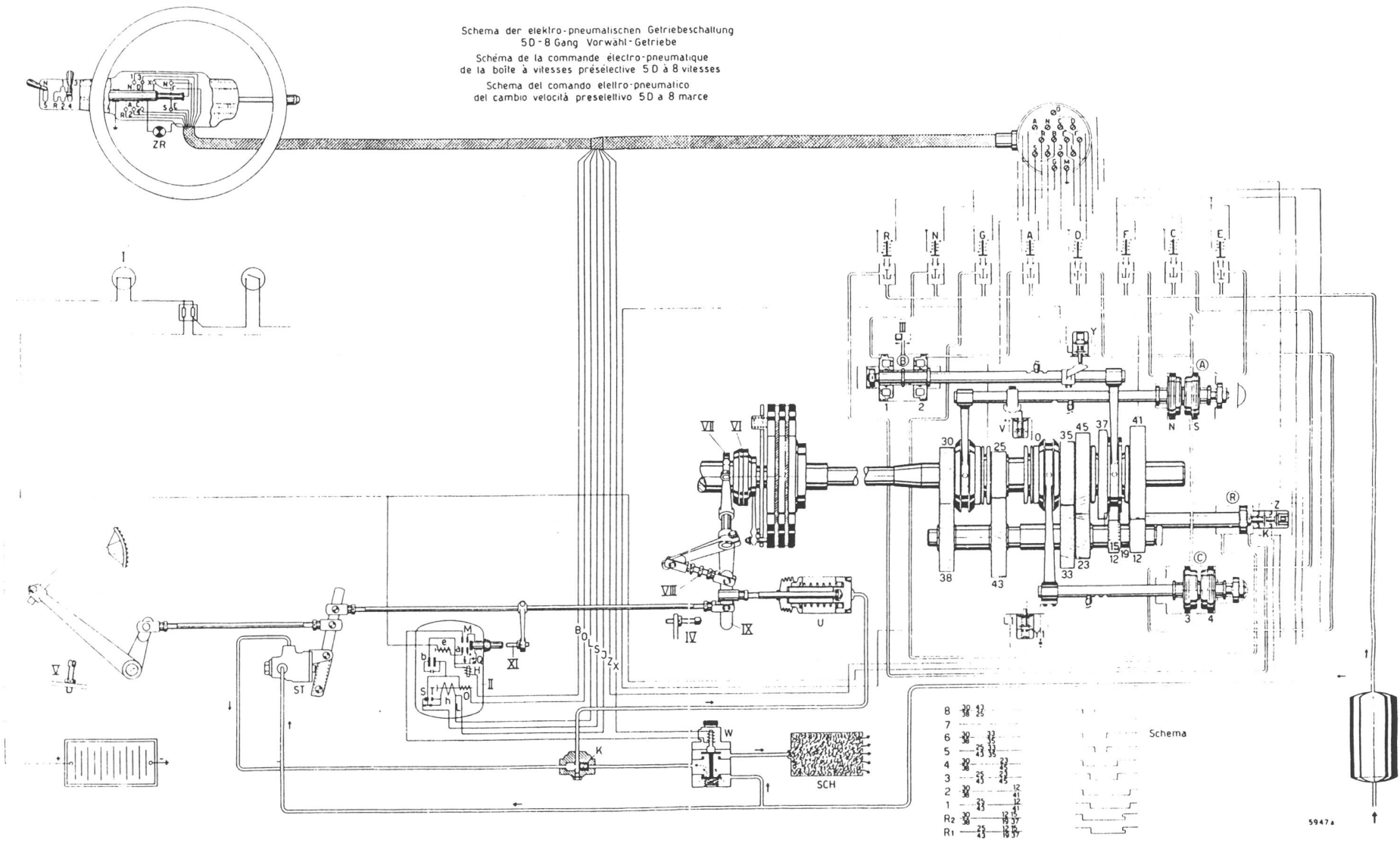
Abb. 48 Schaltschema des 5D-8 Gang-Vorwählgetriebes
