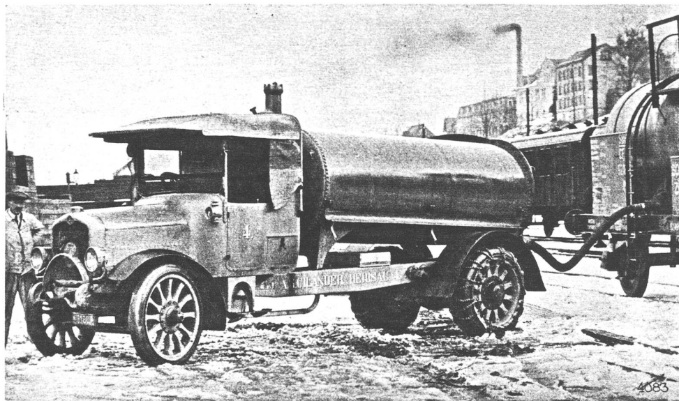
CAMION 5 TONNES AVEC RÉSERVOIR. 5 TONNEN LASTWAGEN MIT ZISTERNE. 5 TON LORRY WITH TANK.
