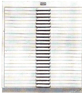
KB 24: Schubladen für schrift- hohe Klischees. Schränk: 1000x900x675 mm Schubladen: 27x795x520 mm Nutzfläche 10 m 2
