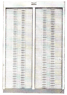
KT 192: 192 Auszüge für unmontierte Klischees. Schränk: 1000x675x675 mm Schieber: 7x270x520 mm Nutzfläche 27 m 2
