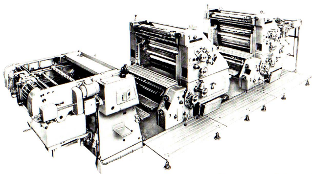
Vierfarben-Offsetpresse Roland-Ultra
