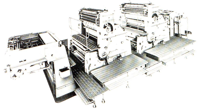
Vierfarben-Offsetpresse Roland-Ultra
