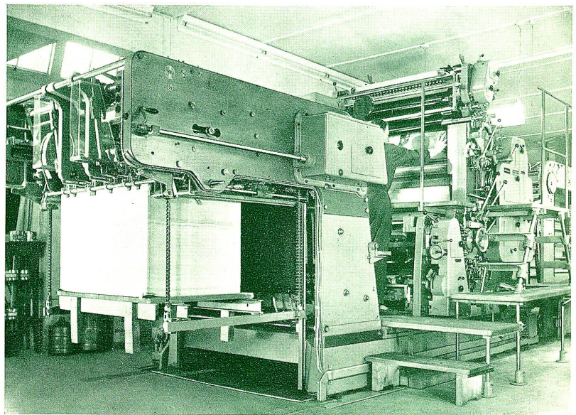
Roland-Ultra IV Zweifarben-Offsetdruckmaschine
