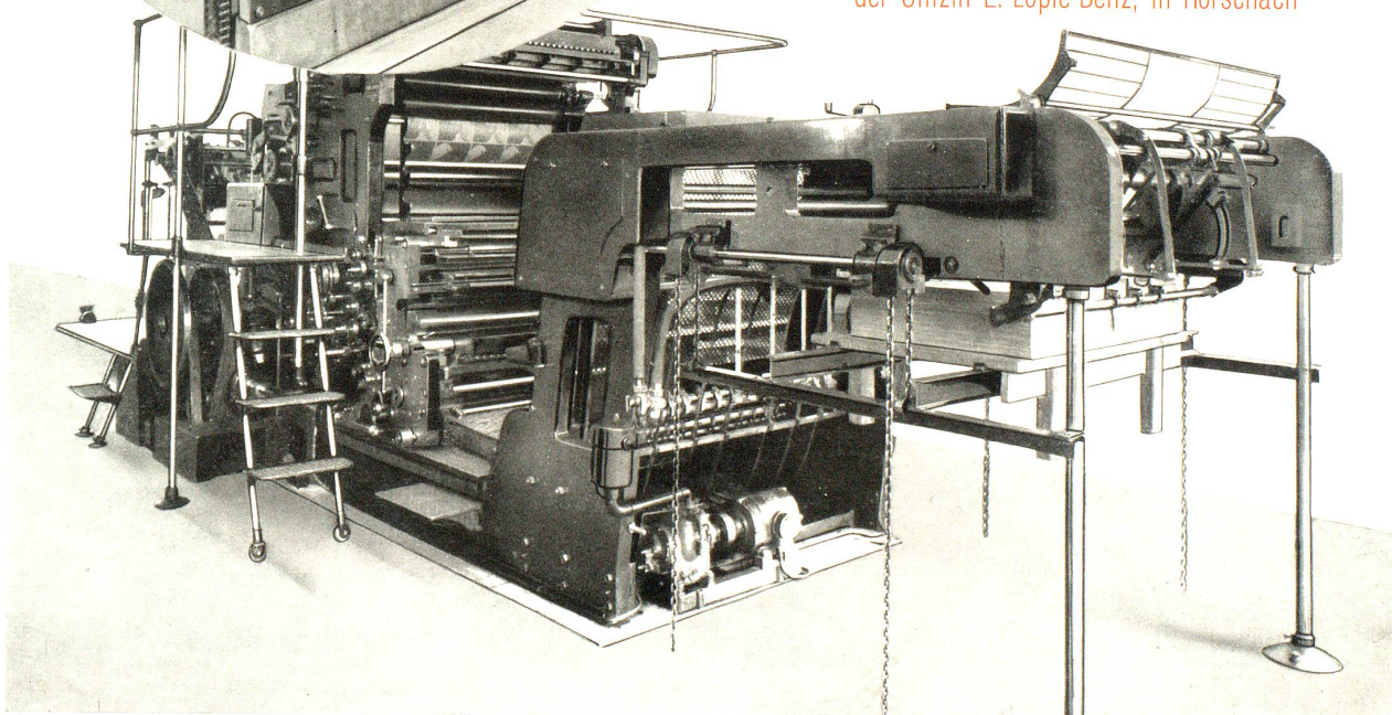
Die Ein- und Mehrfarben-Offset-Druckmaschinen der Offizin E. Löpf-Benz, in Rorschach
