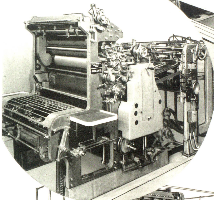
Die Ein- und Mehrfarben-Offset-Druckmaschinen der Offizin E. Löpf-Benz, in Rorschach
