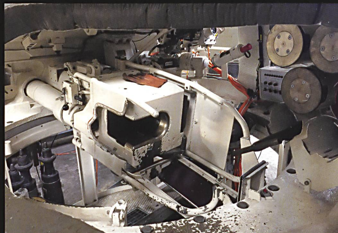
L'intérieur de la tourelle du char Centurion , avec son canon de 10,5 cm rayé.
